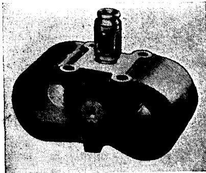
FIG. 19-62.—3J21 magnetron.
